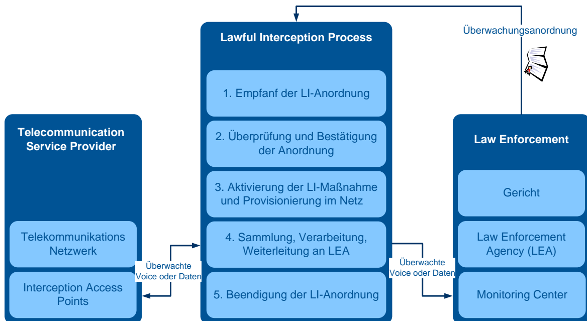
Abbildung 1 : Prozessübersicht Lawful Interception
