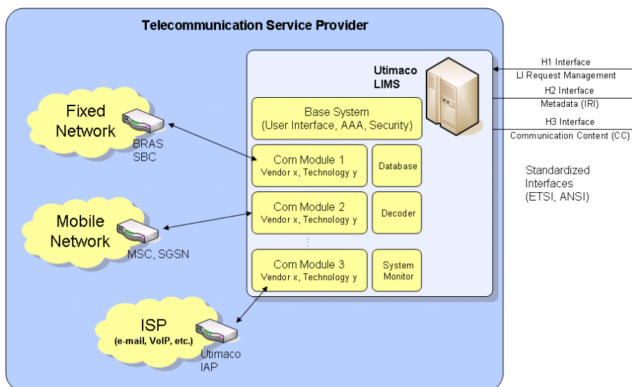
Abbildung 1: Elements von LIMS
