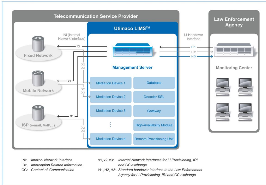
Abbildung 2: Vereinfachte Architektur einer Lawful Interception Lösung
